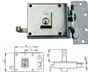
YALE 6 Golpe y llave. Contrapalanca. Caja de 85x120mm. Niquelada.
