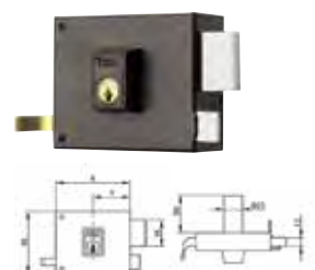
YALE 125 Golpe y llave. Cilindro redondo Ø25mm. Caja de 85x125mm. Pintada.
