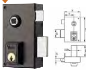
YALE 56B Golpe y llave. Cilindro redondo Ø25mm. Nueca para manilla. Caja de 60x112mm. Pintada.
