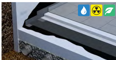
Solera amb barrera de radó Sistema RAD3 180-40 P Elast
