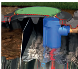
Depuradora one2clean amb cúpula micro
